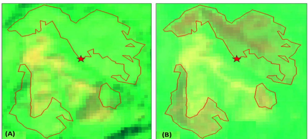
Hình 6. Các vùng mất rừng tại tọa độ 22°15'25''B - 102°15'45''Đ
