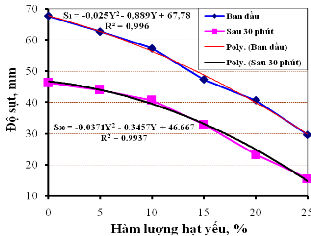
Hình 01. Quan hệ hàm lượng hạt yếu và độ sụt
