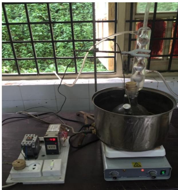
Hình 01. Thiết bị hoá lỏng bột gỗ
